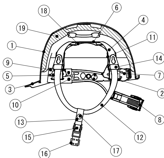
断面図
